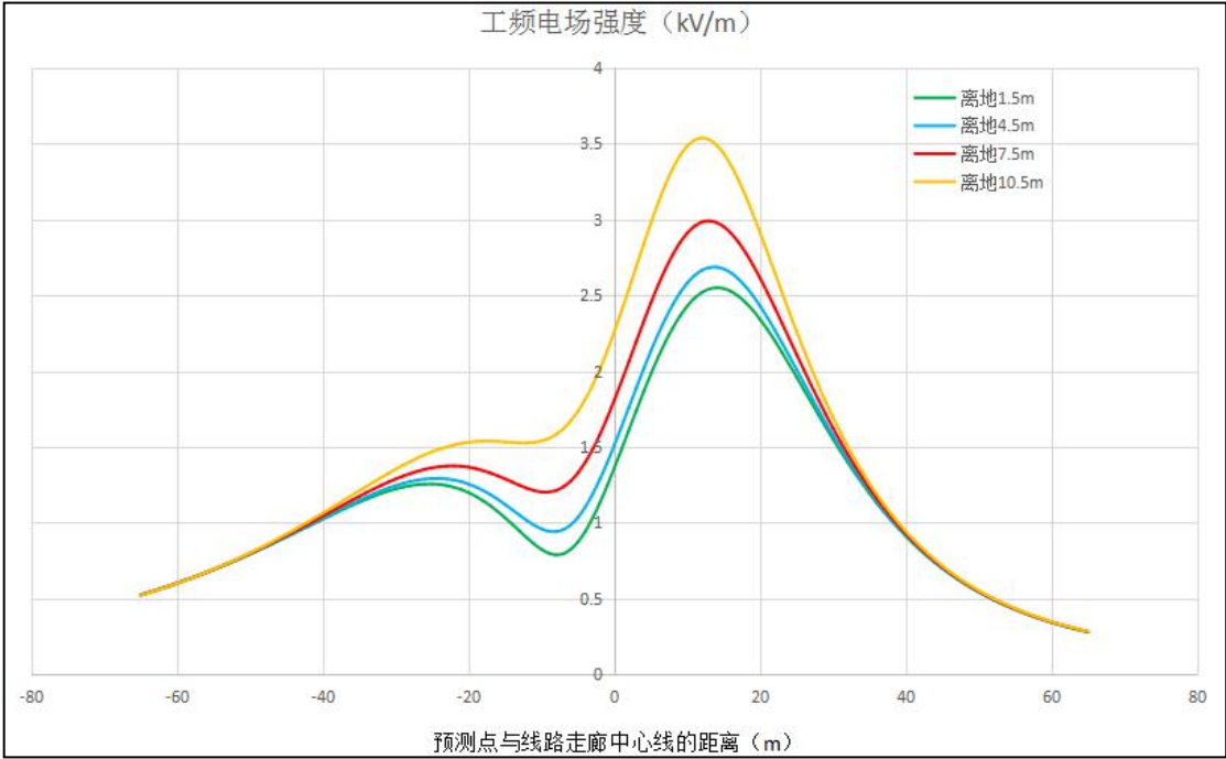
图 6-4 项目导线对地高度为 14m 时线下工频电场强度分布曲线图
