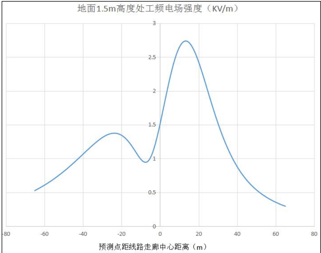
图 6-7 重新紧线段 500kV 输电线路工频电场分布曲线
