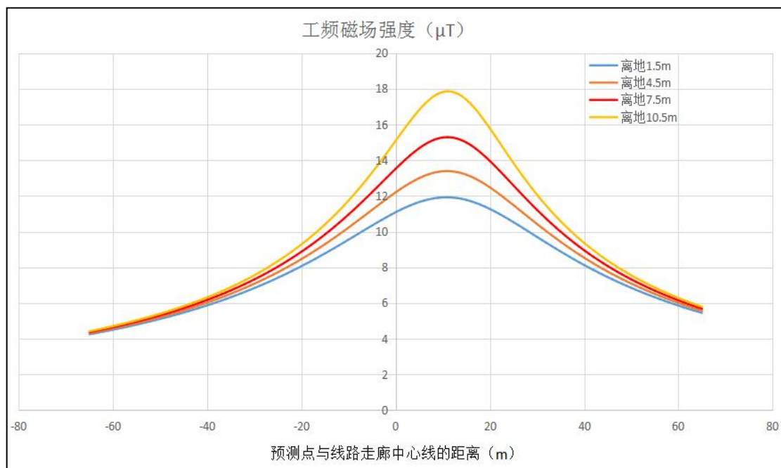
图 6-6 项目导线对地高度为 25.4m 时线下工频磁场强度分布曲线
