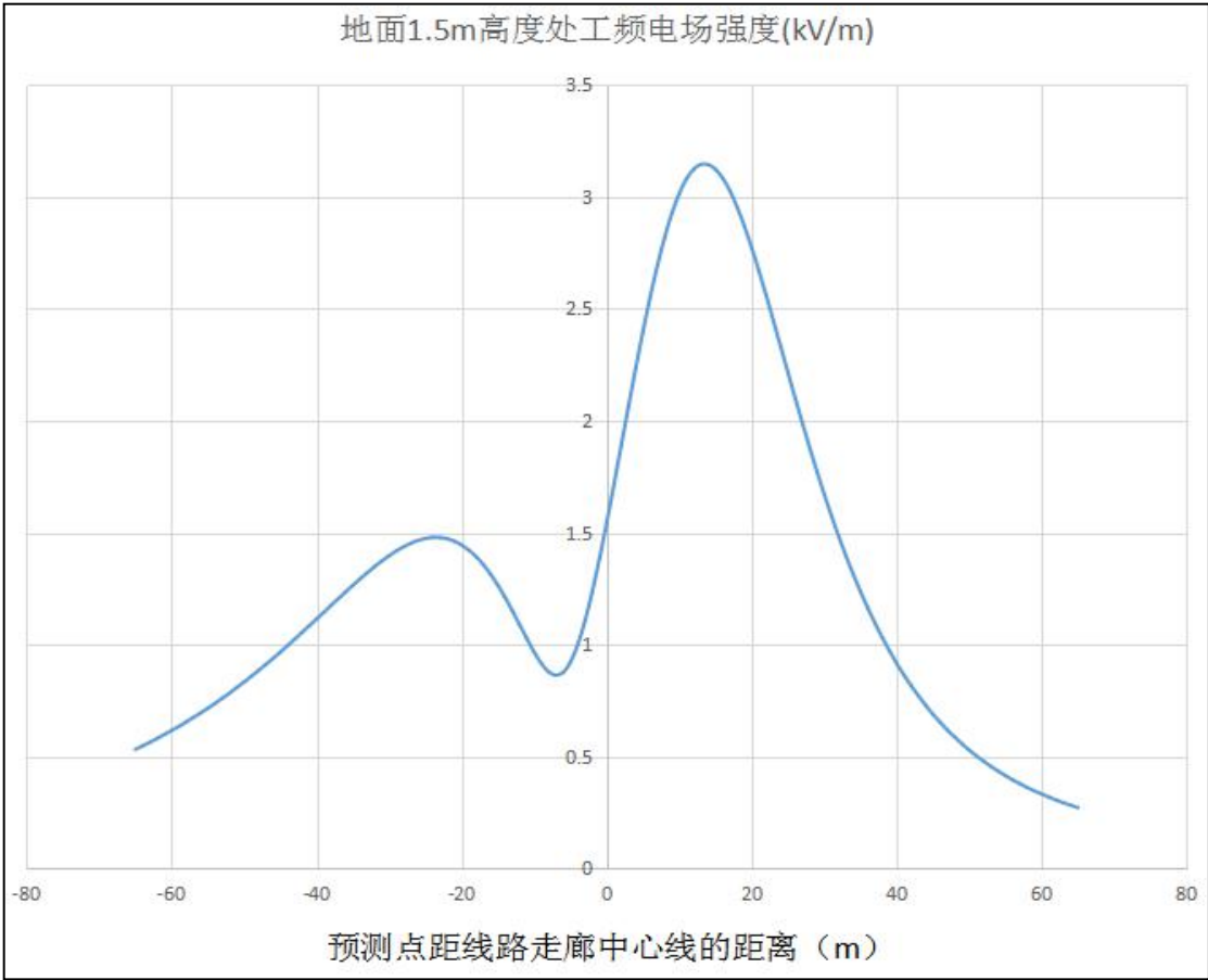
图 6-3 项目导线对地高度为 22.4m 时线下工频电场强度分布曲线
