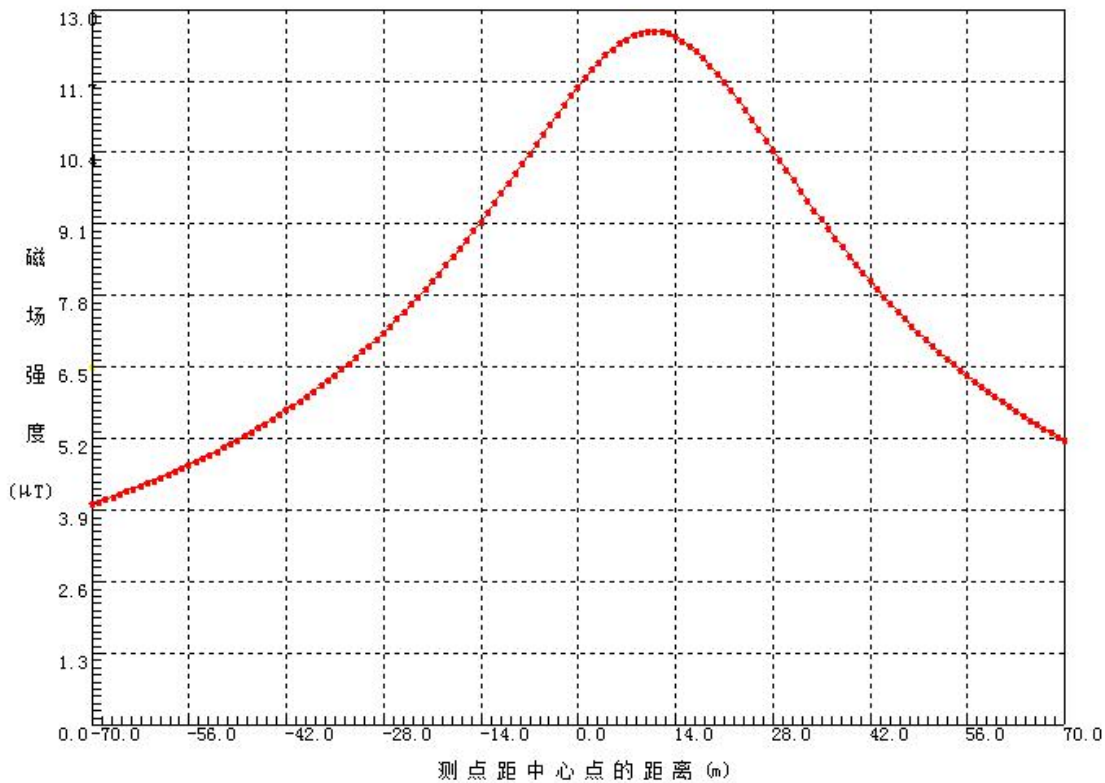
图 6-8 重新紧线段 500kV 输电线路工频磁感应强度分布曲线
