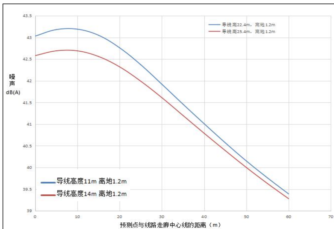
图 6-9 项目线路噪声影响趋势图
