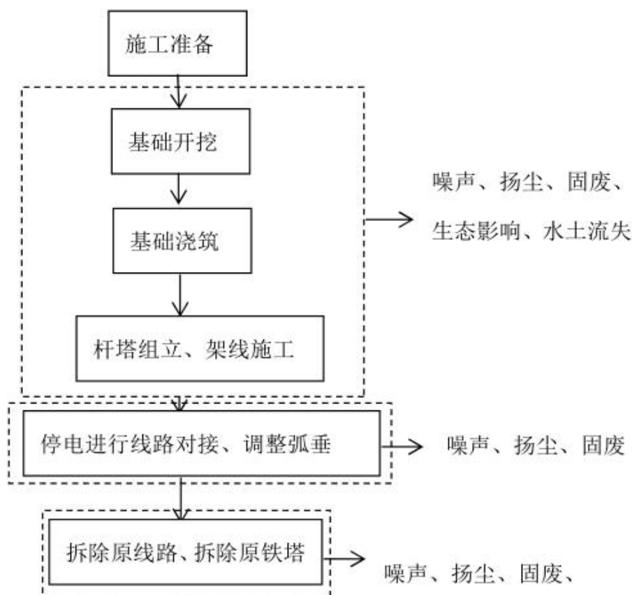
图 3-6 施工期工序流程及产污位置图
