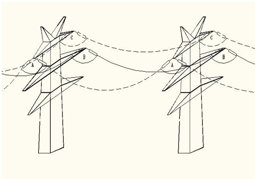
图 3-4 项目相序示意图
