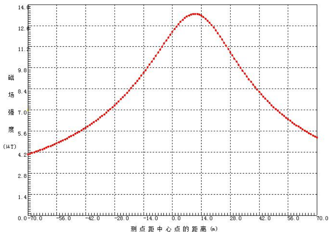
图 6-5 项目导线对地高度为 22.4m 时线下工频磁场强度分布曲线
