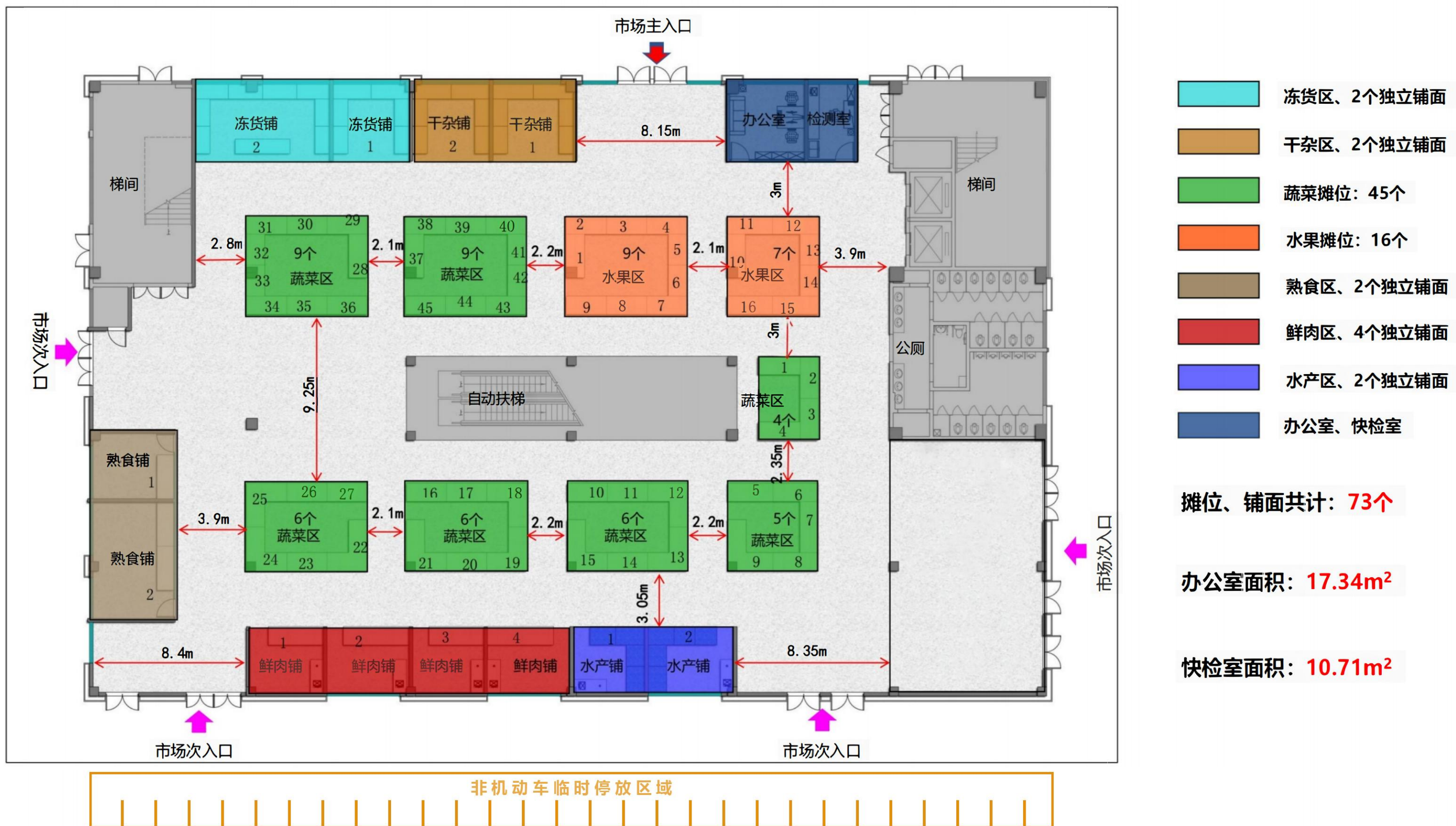
桃花山购物广场摊店平面图
